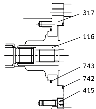
SAE 'B' & 'BB' T/D KIT
