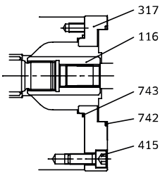
SAE 'BB' T/D KIT
